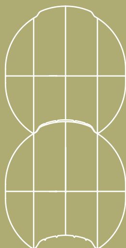
Круглые клееные бревна (MRL) Ø 226 Ø 260
